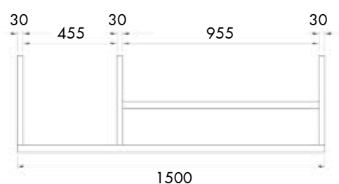
Dimensioni per tavolo 1500 mm
