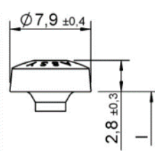
Testa cilindrica
