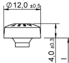
Testa cilindrica
