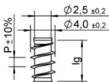
Filettatura sottotesta Lg2 < 4 \times d , P = 1,8; 2,6; 3,6
