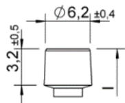
Testa cilindrica
