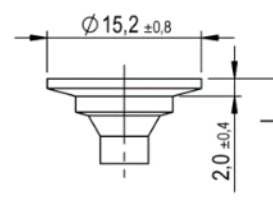
Testa a rondella larga/testa a bottone II - con e senza bombatura
