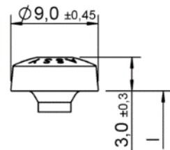
Testa cilindrica
