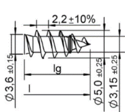
Filettatura semplice
