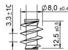
Filettatura sottotesta tipo P
