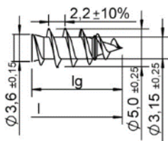
Filettatura semplice
