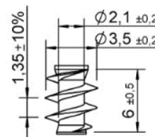
Filettatura sottotesta
