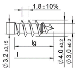
Legno duro
