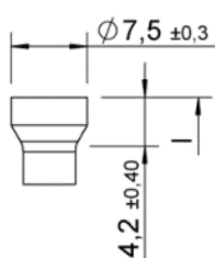
Testa cilindrica piccola
