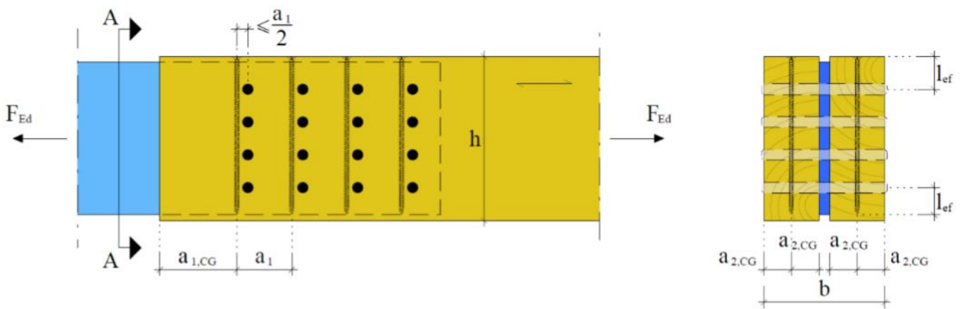
Figura A.6.1 unione acciaio-legno con perni di centratura e legni laterali rinforzati alla trazione trasversale
