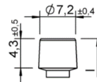
Testa cilindrica
