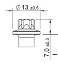
Testa rotonda esagonale esterna – con e senza rondella
