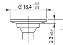
Testa a rondella larga/testa a bottone II – con e senza bordi fresati
