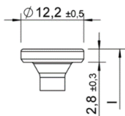
Testa piatta
