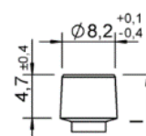
Testa cilindrica
