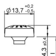
Testa cilindrica
