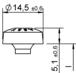
Testa cilindrica
