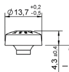
Testa cilindrica
