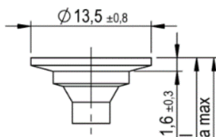
Testa a rondella larga/testa a bottone II
